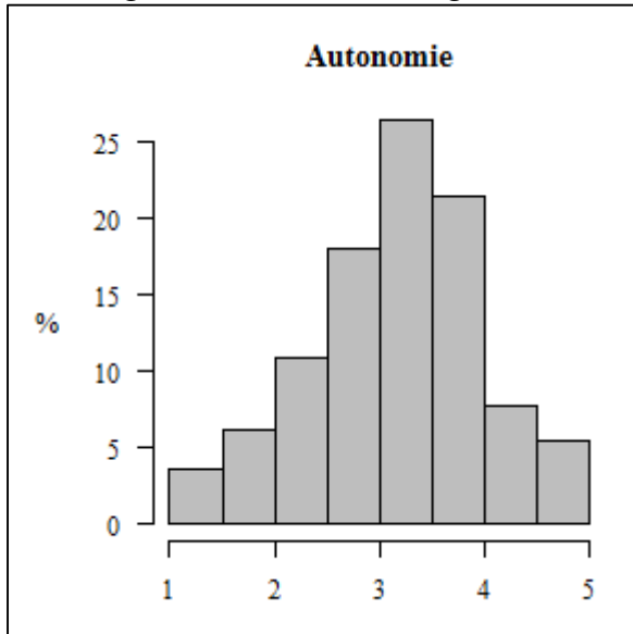
Abbildung 15: Autonomie – Histogramm
