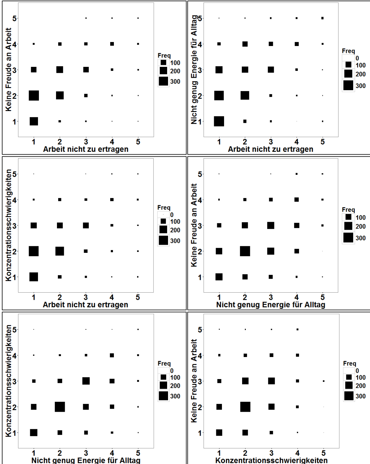
Abbildung 68: Burnout – Streudiagramm-Plots
