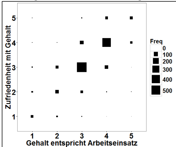
Abbildung 30: Einkommen – Streudiagramm-Plot
