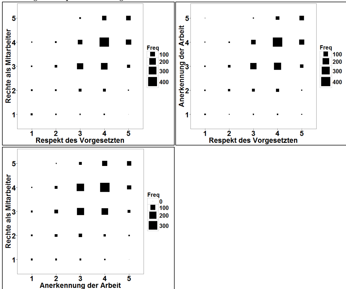
Abbildung 59: Respekt – Streudiagramm-Plots
