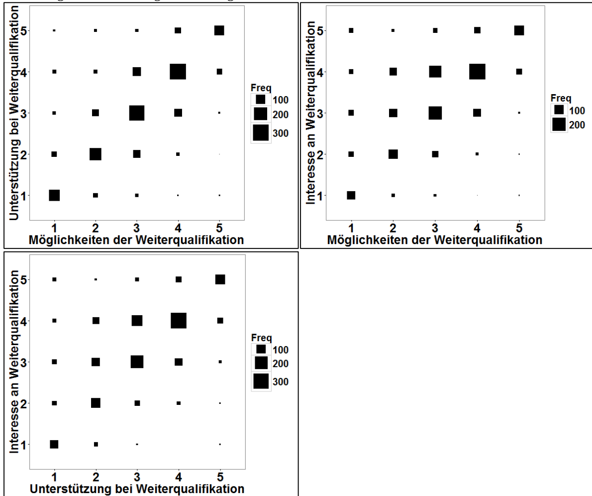
Abbildung 33: Ausbildung – Streudiagramm-Plots
