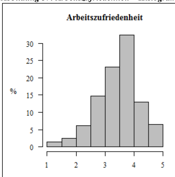
Abbildung 57: Arbeitszufriedenheit – Histogramm
