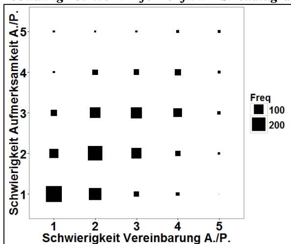
Abbildung 73: Work-Life-Konflikt – Streudiagramm-Plot
