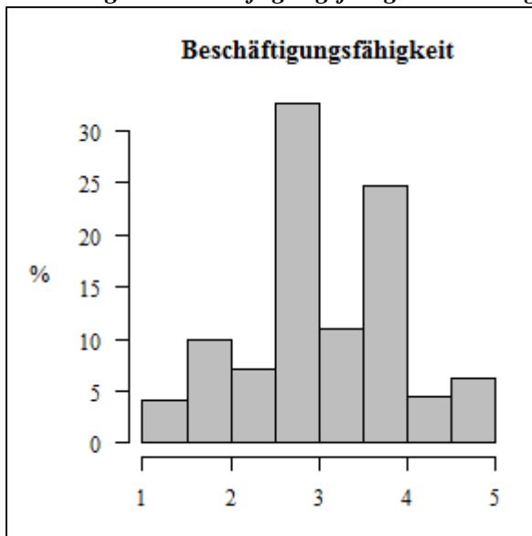
Abbildung 41: Beschäftigungsfähigkeit – Histogramm
