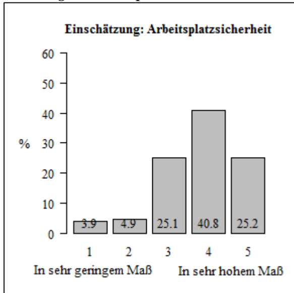
Abbildung 38: Arbeitsplatzsicherheit – Balkendiagramme
