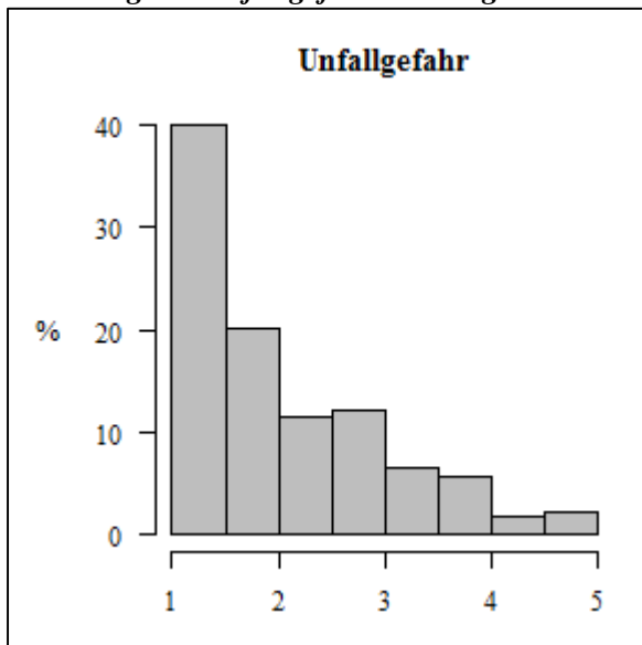
Abbildung 50: Unfallgefahr – Histogramm
