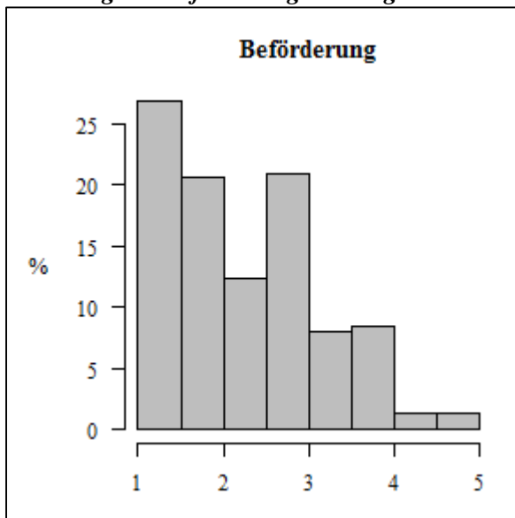
Abbildung 37: Beförderung – Histogramm
