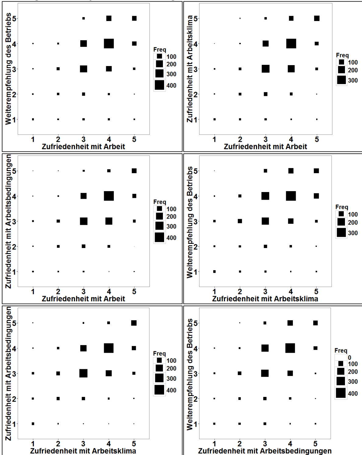
Abbildung 56: Arbeitszufriedenheit – Streudiagramm-Plots
