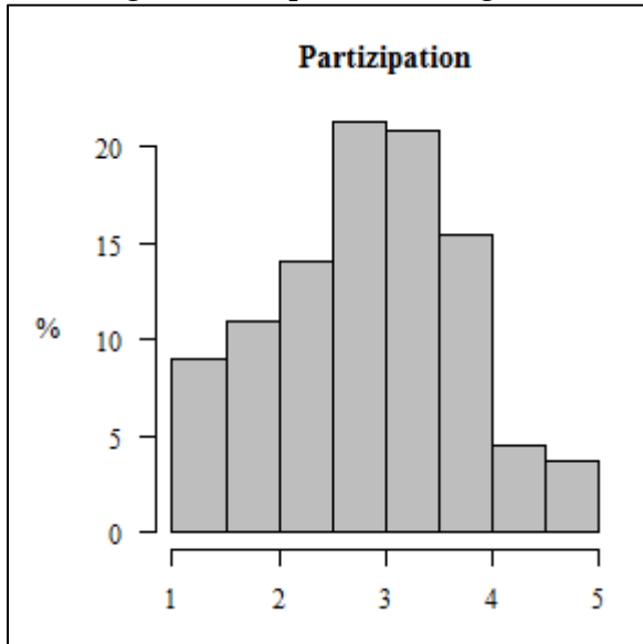
Abbildung 9: Partizipation – Histogramm
