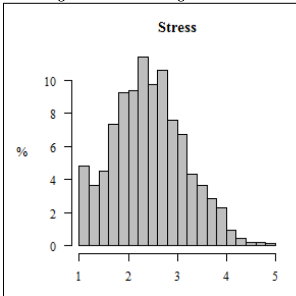
Abbildung 66: Stress – Histogramm
