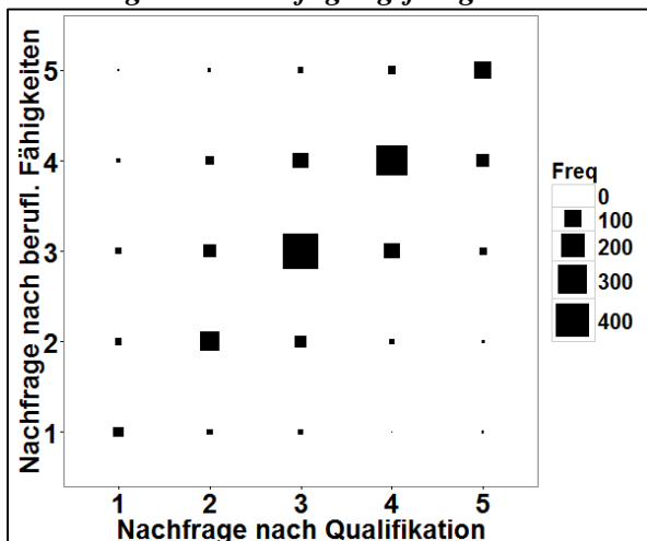
Abbildung 40: Beschäftigungsfähigkeit – Streudiagramm-Plot
