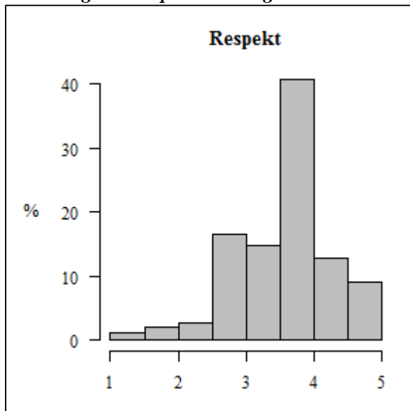
Abbildung 60: Respekt – Histogramm
