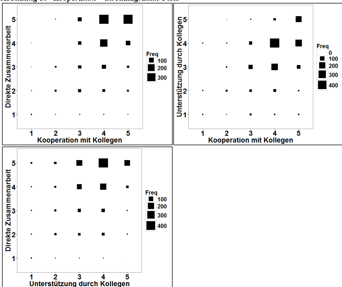
Abbildung 5: Kooperation – Streudiagramm-Plots
