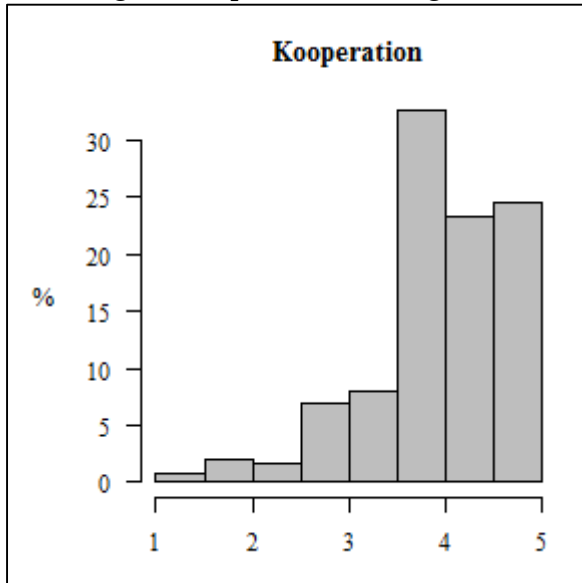
Abbildung 6: Kooperation – Histogramm
