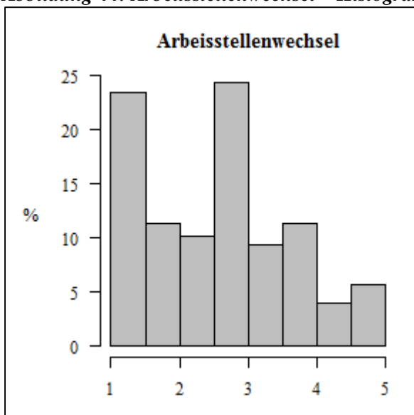
Abbildung 44: Arbeitsstellenwechsel – Histogramm
