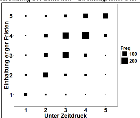
Abbildung 20: Zeitdruck – Streudiagramm-Plot
