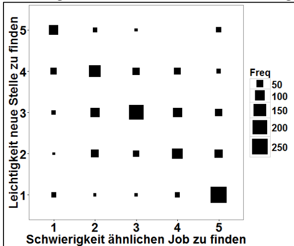
Abbildung 43: Arbeitsstellenwechsel – Streudiagramm-Plot
