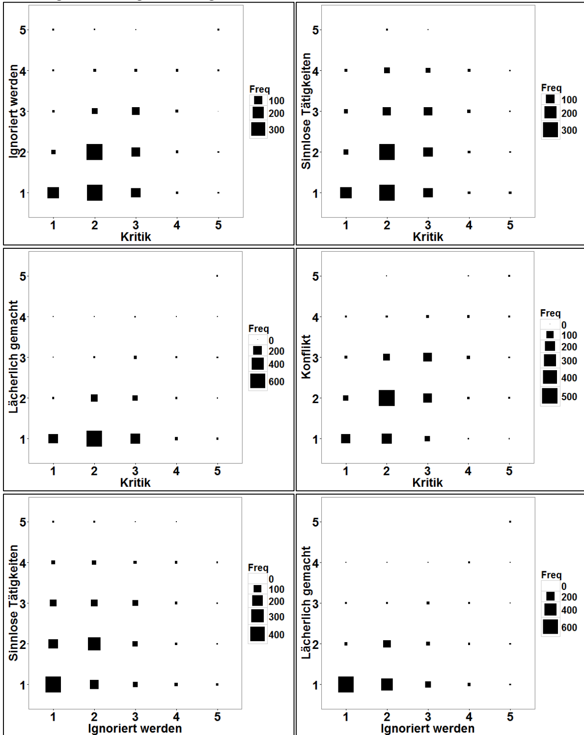
Abbildung 23: Mobbing – Streudiagramm-Plots
