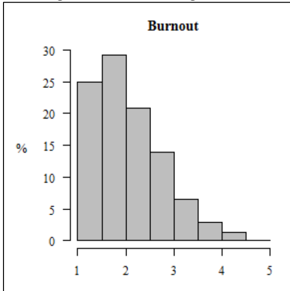
Abbildung 69: Burnout – Histogramm
