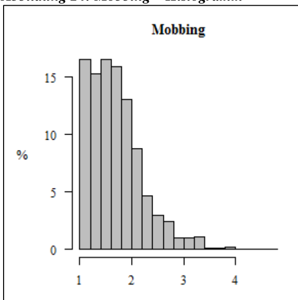
Abbildung 24: Mobbing – Histogramm
