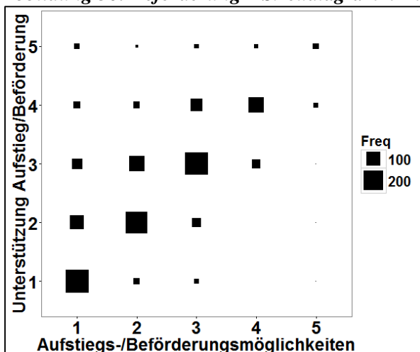
Abbildung 36: Beförderung – Streudiagramm-Plot
