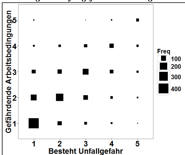
Abbildung 49: Unfallgefahr – Streudiagramm-Plot
