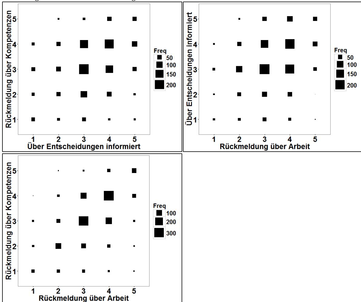
Abbildung 11: Feedback – Streudiagramm-Plots
