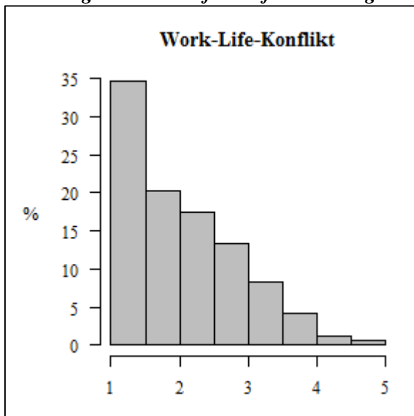
Abbildung 74: Work-Life-Konflikt – Histogramm
