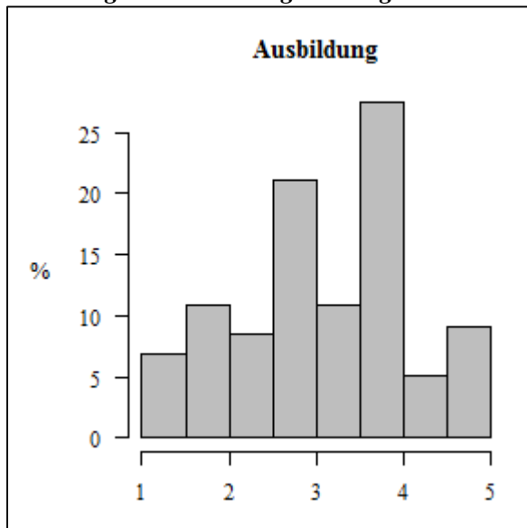
Abbildung 34: Ausbildung – Histogramm
