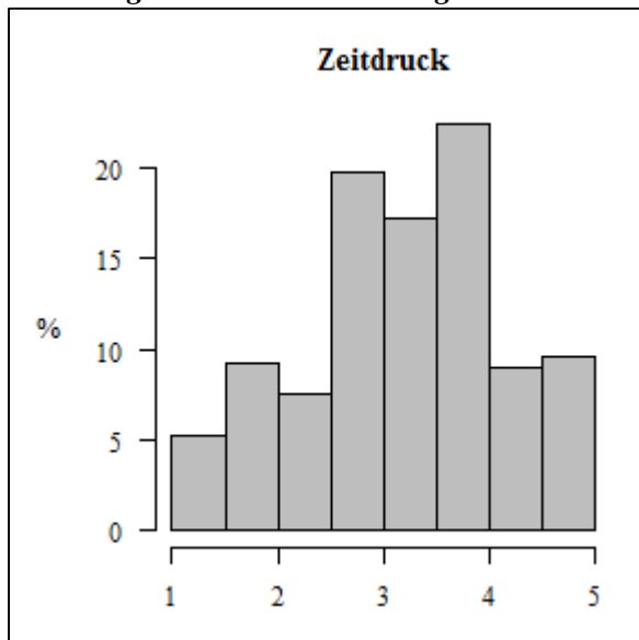
Abbildung 21: Zeitdruck – Histogramm
