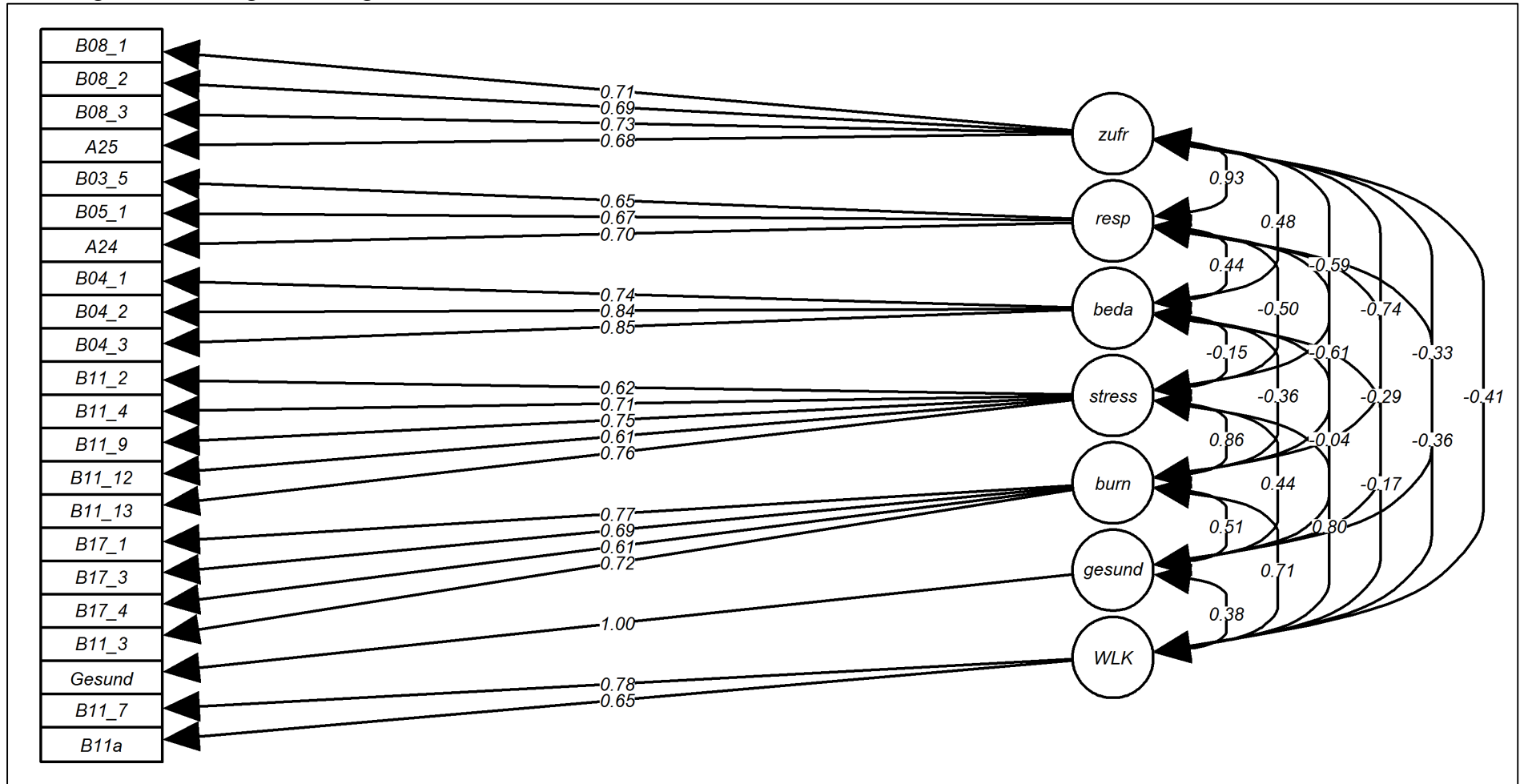
Abbildung 77: Well-Being: KFA-Diagramm
