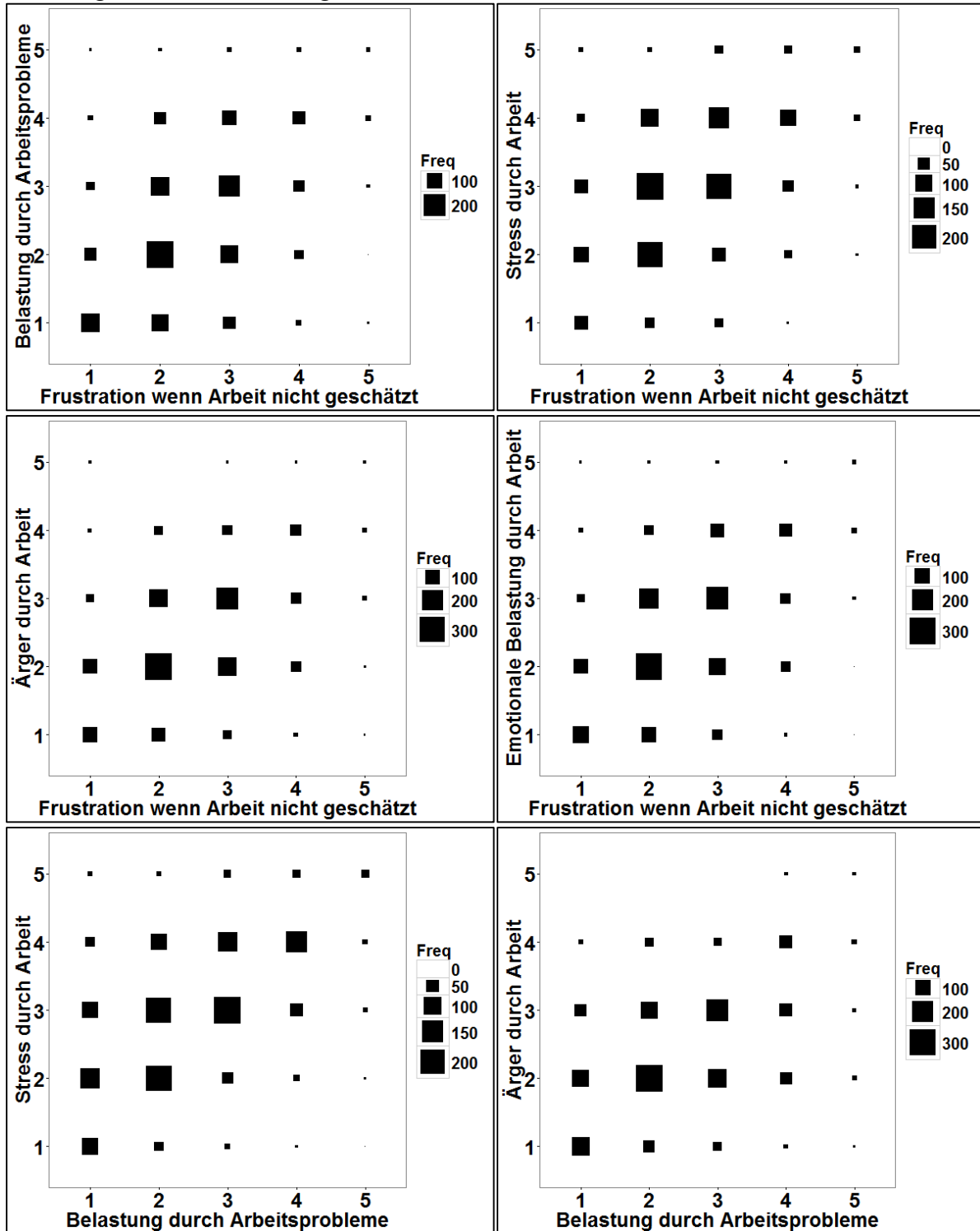
Abbildung 65: Stress – Streudiagramm-Plots
