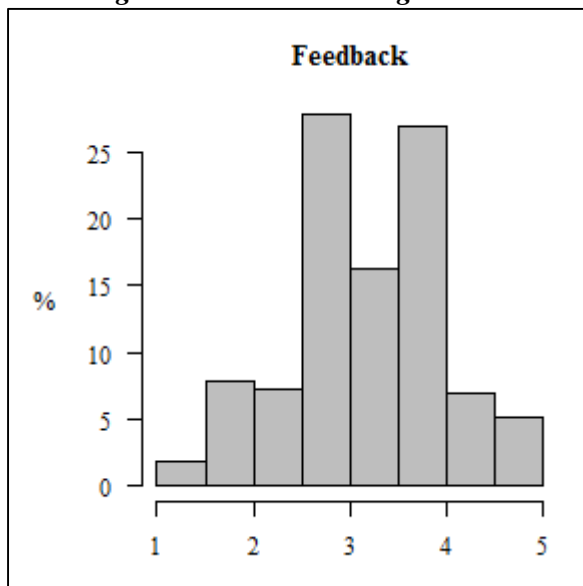
Abbildung 12: Feedback – Histogramm
