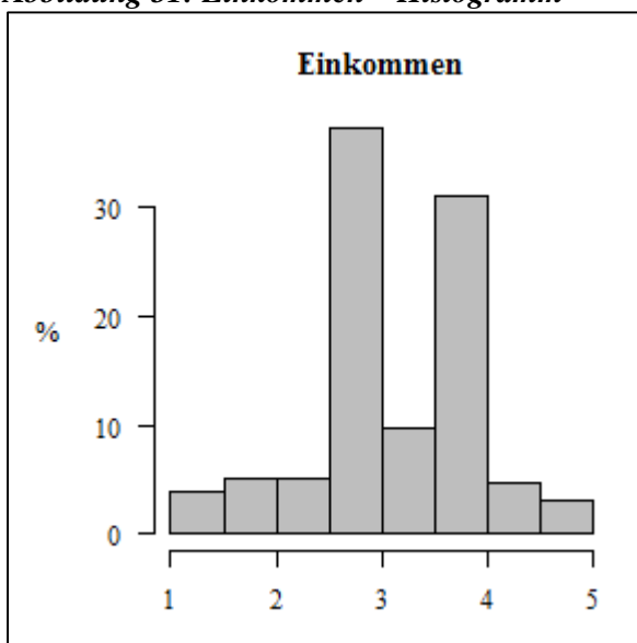
Abbildung 31: Einkommen – Histogramm
