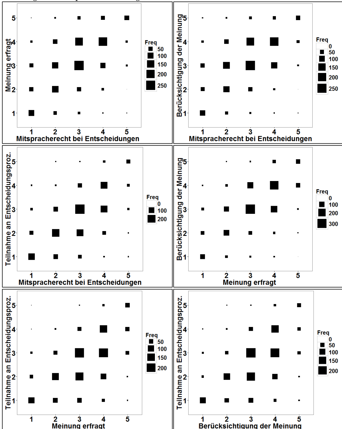
Abbildung 8: Partizipation – Streudiagramm-Plots
