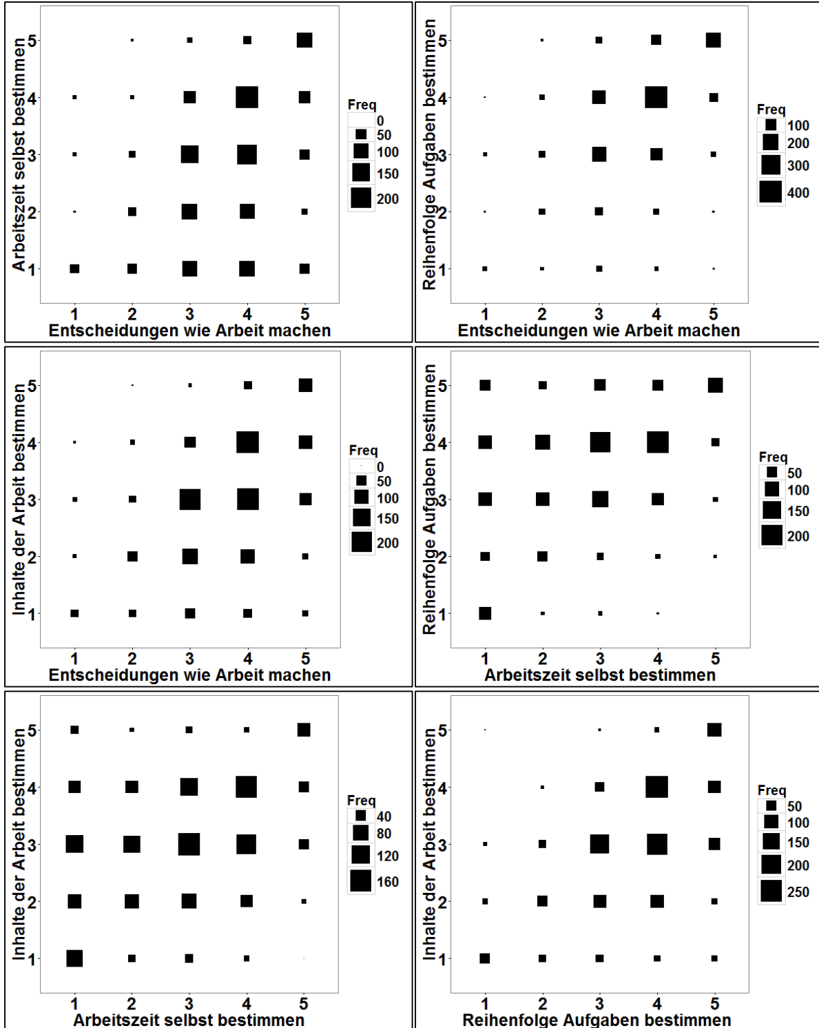
Abbildung 14: Autonomie – Streudiagramm-Plots
