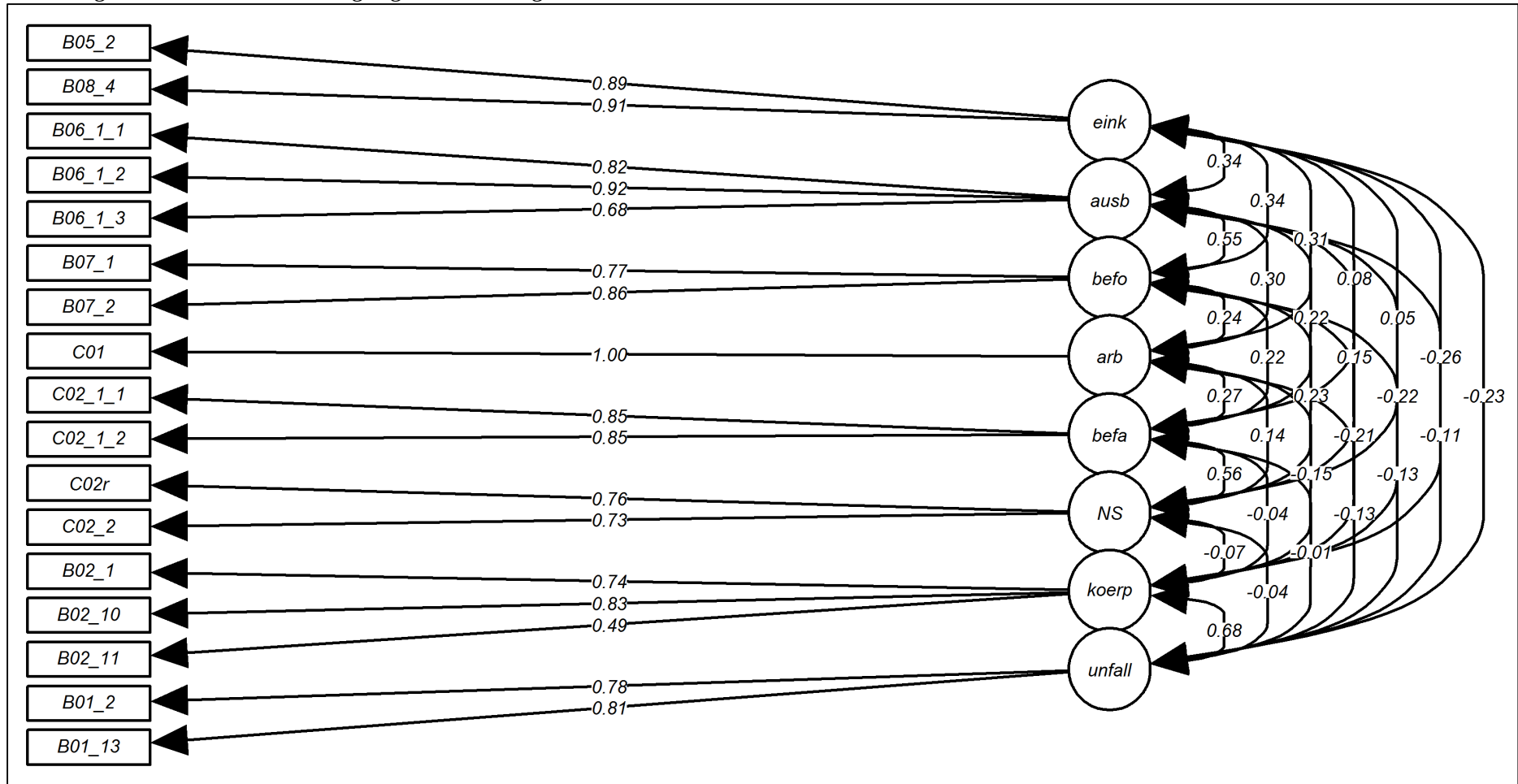
Abbildung 53: Arbeitsrahmenbedingungen: KFA-Diagramm
